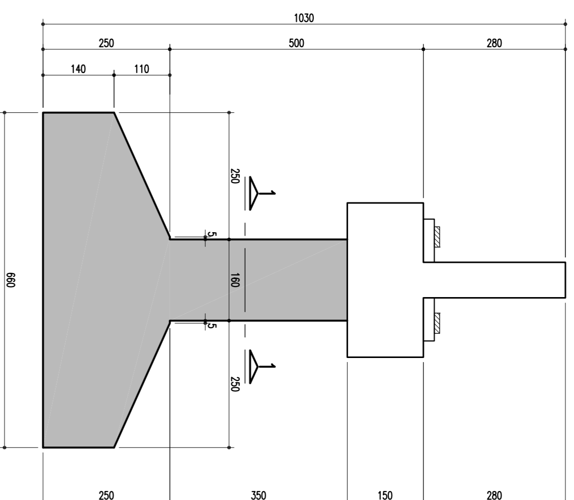
ELEVAÇÃO EM CORTE A-A (P49 = 5,00m) ESCALA = 1/75
