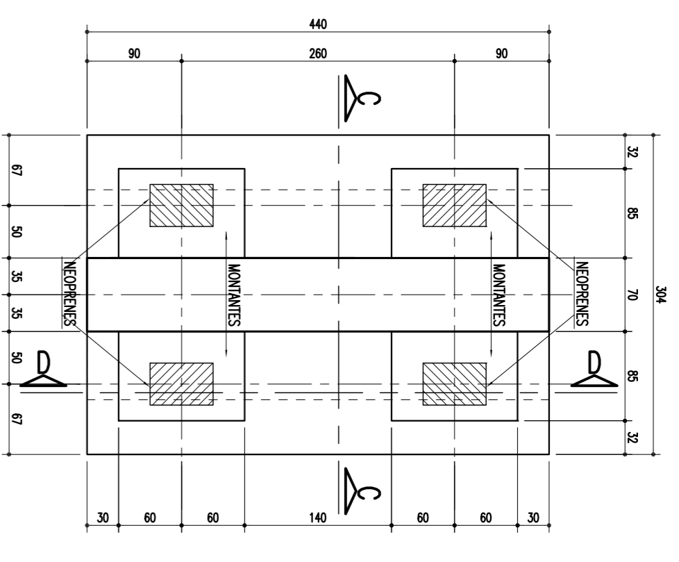
DETALHE: TRAVESSA E LOGAÇÃO DOS MONTANTES-85/120/21.5 ESCALA = 1/50
