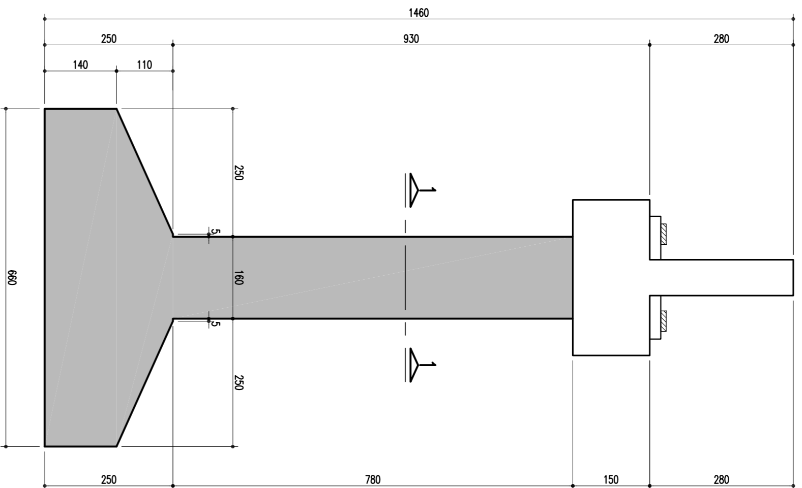
ELEVAÇÃO EM CORTE A-A (P47 = 9,30m) ESCALA = 1/75
