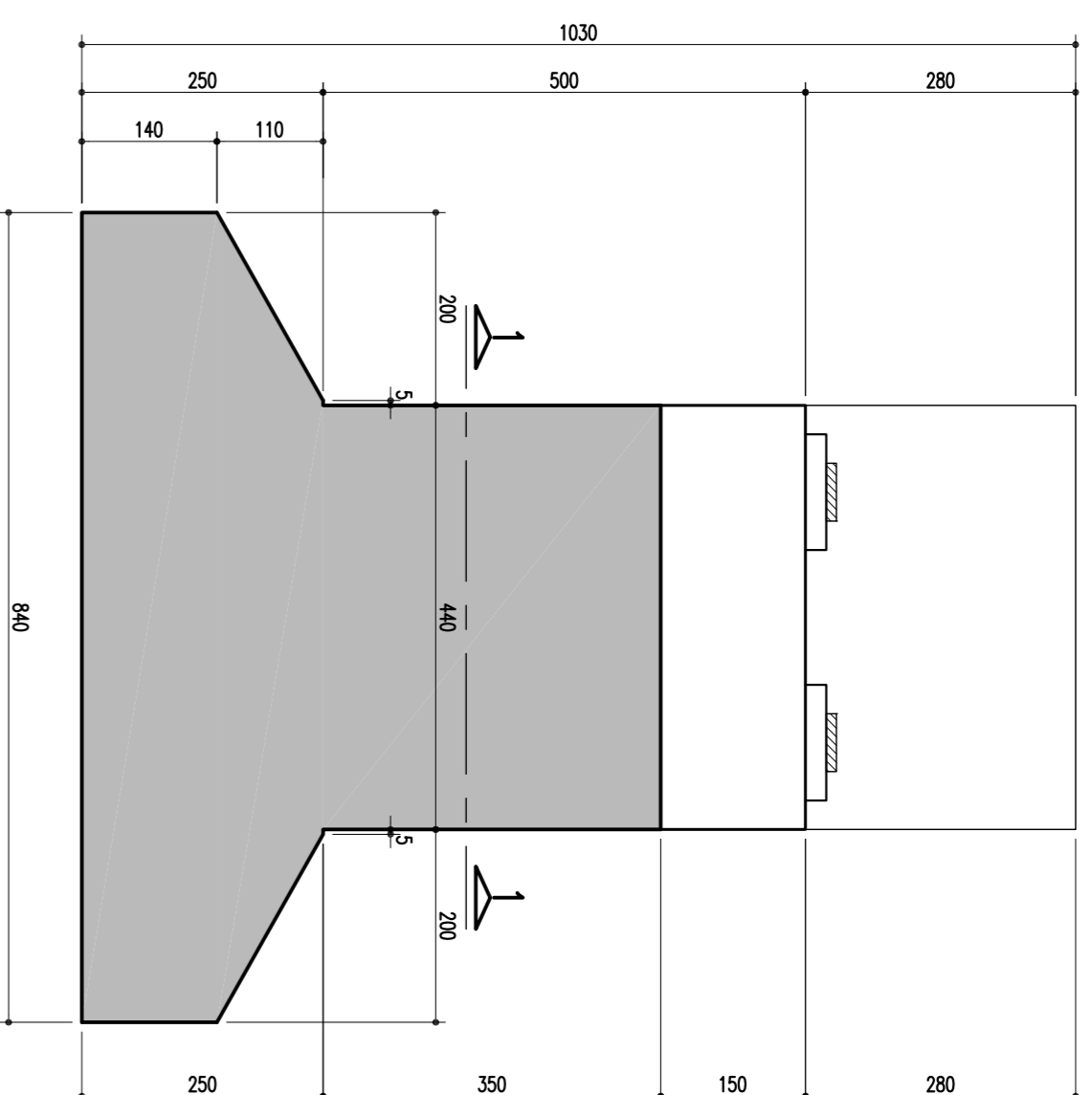
ELEVAÇÃO EM CORTE B-B (P49 = 5,00m) ESCALA = 1/75
