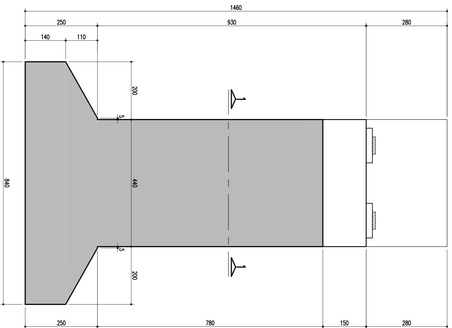
ELEVAÇÃO EM CORTE B-B (P47 = 9,30m) ESCALA = 1/75
