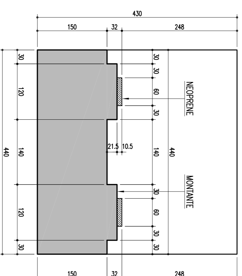
TRAVESSA - CORTE D-D ESCALA = 1/30
