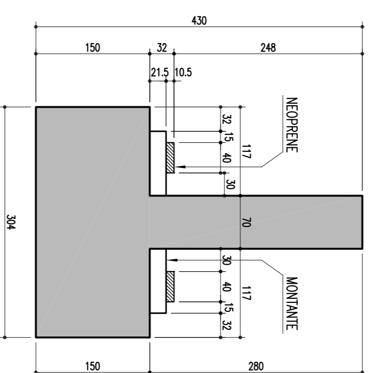
TRAVESSA - CORTE C-C ESCALA = 1/30
