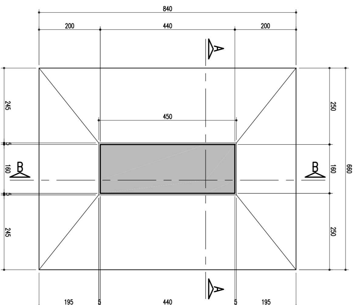
SAPATAS - P47/P48 E P49 - 660/840 ESCALA = 1/75
