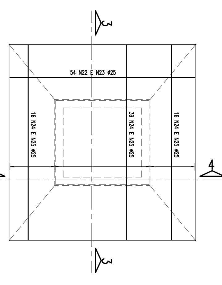
ARMADÃO DA SAPATA - 1000/1040 - P07 E P28
