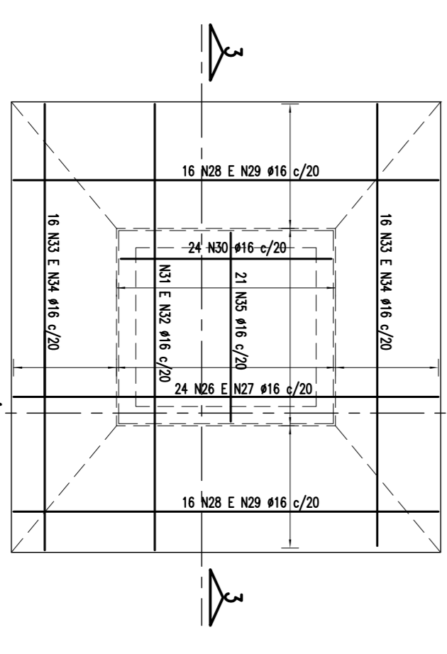
ARMADÃO DA SAPATA - 1000/1040 - P07 E P28
