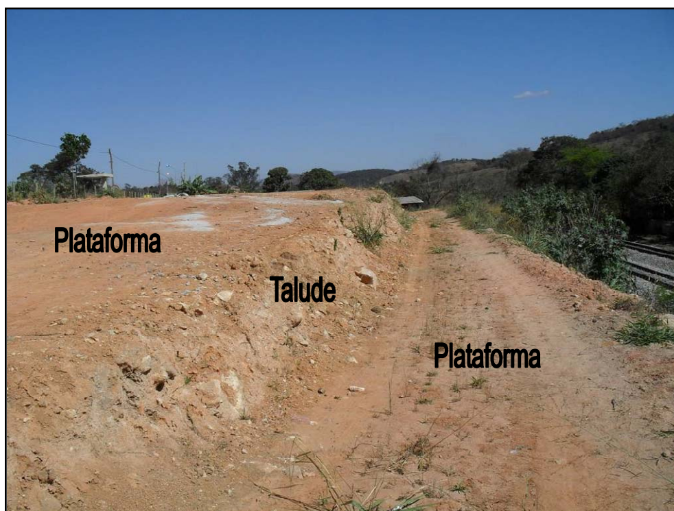
Foto 7 - Plataforma e talude a serem recuperados na área de ampliação do Pátio Ferroviário de Vianópolis.
