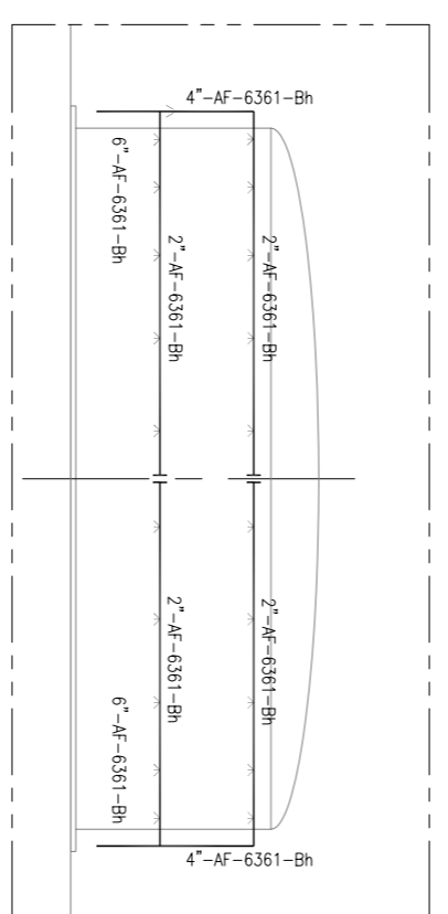
ELEVACÃO TIPO ANEIS DE ASPERSORES
