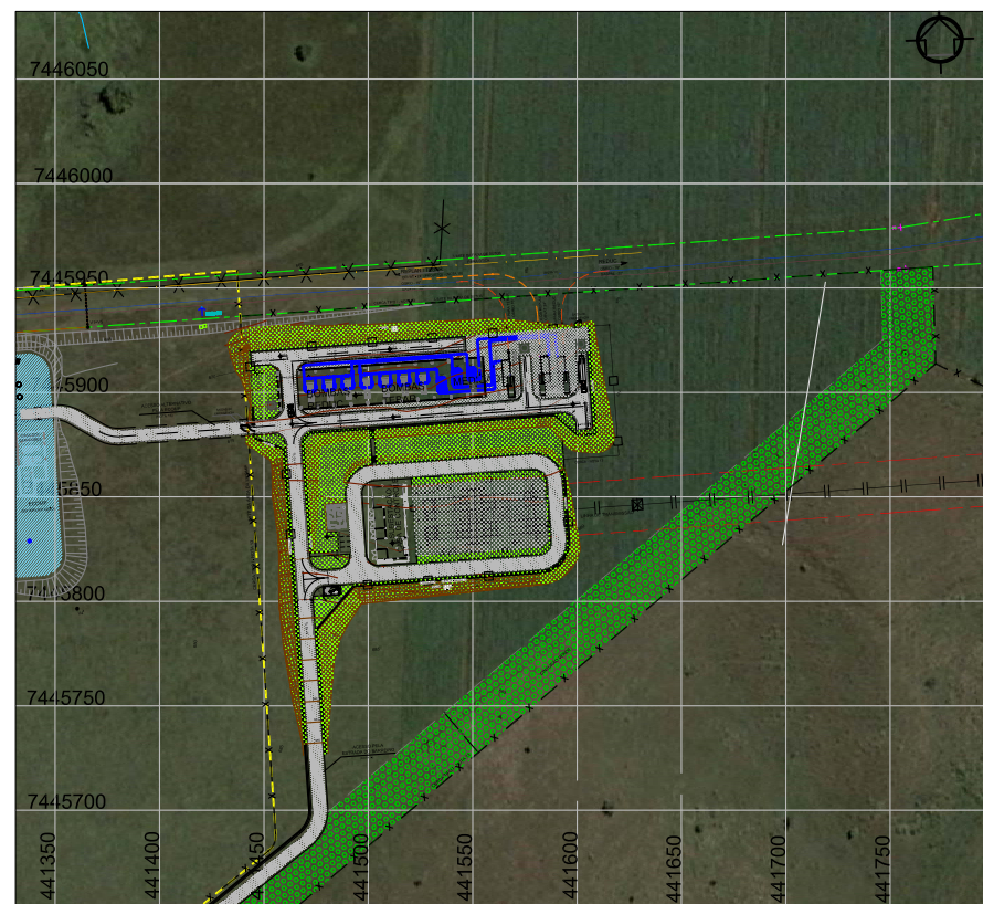
LAY OUT DA ESTAÇÃO DE BOMBEAMENTO DE TAUBATÉ EM IMAGEM DE SATÉLITE Escala 1:4.000
