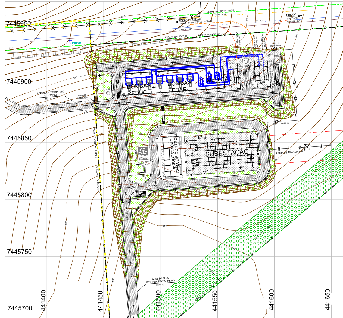
DETALHE DO LAY OUT DA ESTAÇÃO DE BOMBEAMENTO DE TAUBATÉ Escala 1:2.000
