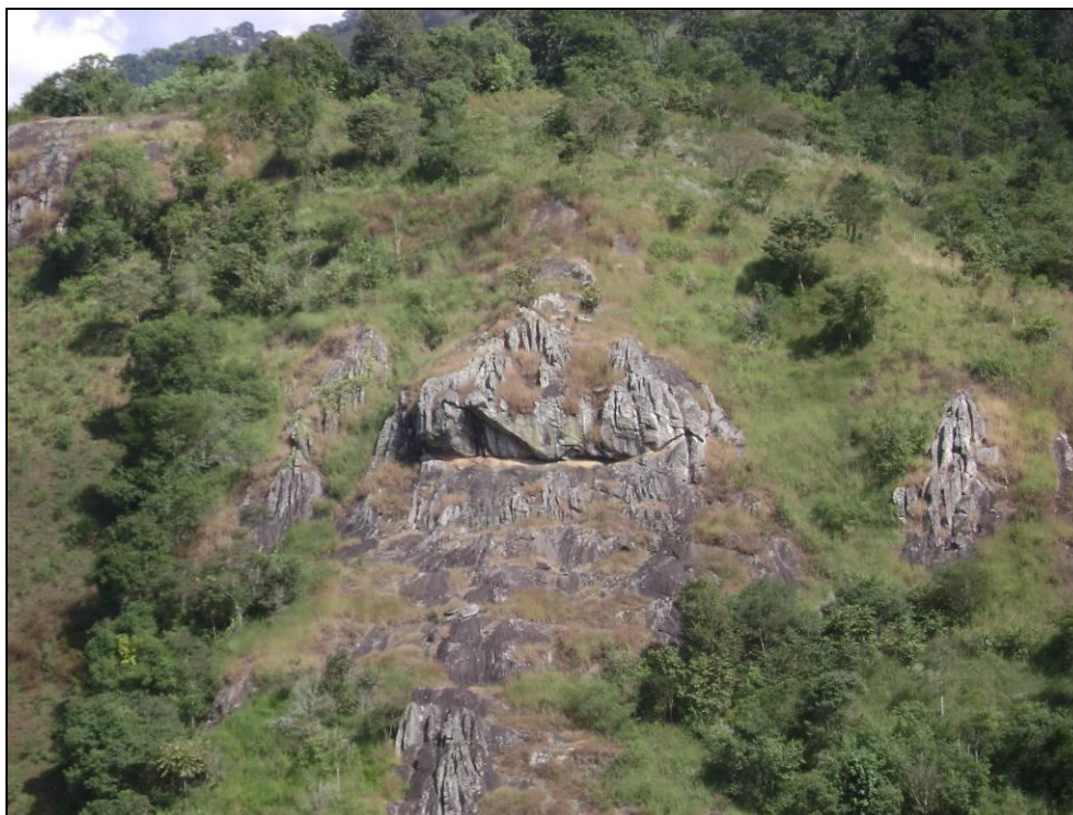
Foto 01 - Lâpias desenvolvidos de acordo com o Sn da rocha. MG-482, próximo à localidade de Pé do Morro, município de Itaverava (Coord. UTM 23 K 637.934/7.715.039).
