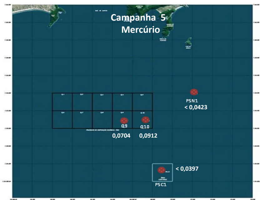
Figura 4.3-5. Variação espacial da concentração de mercúrio (mg/kg) das amostras coletadas na Campanha 5.
