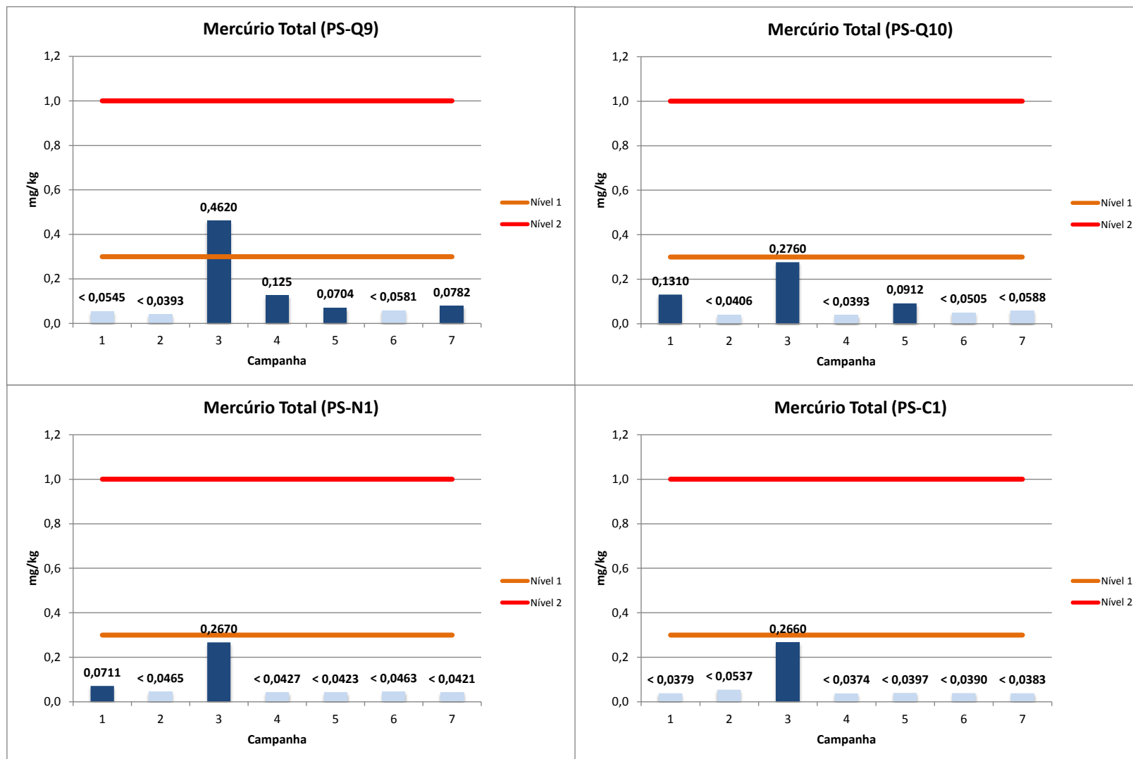
Figura 4.1-1. Concentração de mercúrio nas amostras de sedimentos coletadas nas quadrículas Q-9 e Q-10 (PS-Q9 e PS-Q10), no ponto a nordeste do PDO (PS-N1) e na área a ser controlada (PS-C1), referentes às Campanhas 1 a 7.
