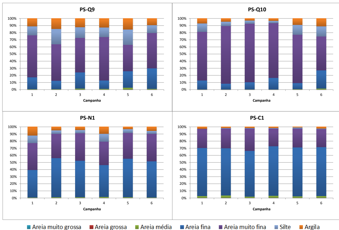
Figura 4.2-1. Composição granulométrica do sedimento das amostras PS-Q9, PS-Q10, PS-N1 e PS-C1 das Campanhas 1 a 6.
