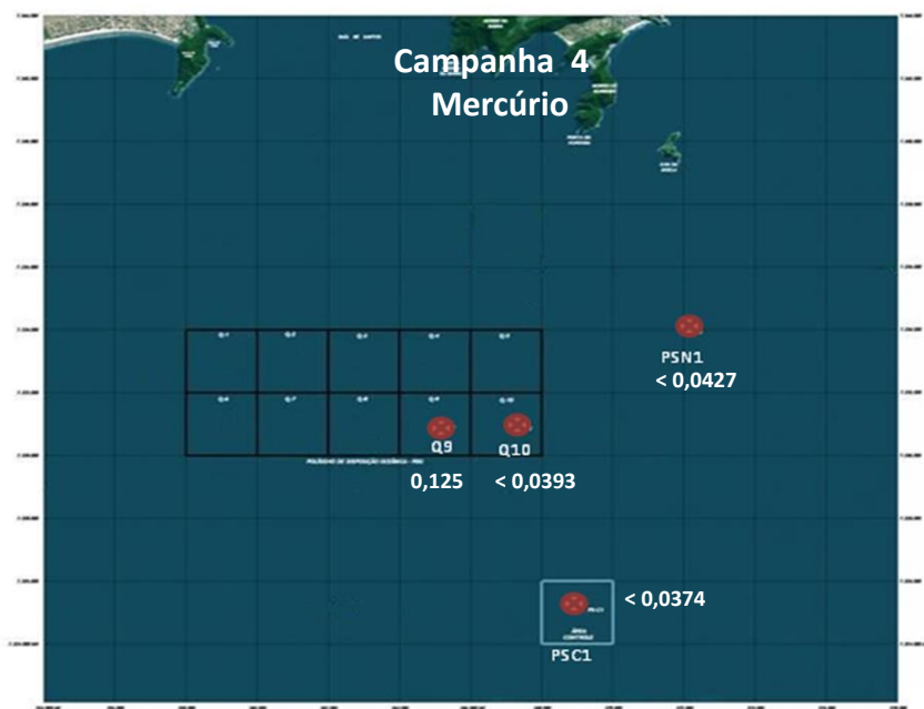
Figura 4.3-4. Variação espacial da concentração de mercúrio (mg/kg) das amostras coletadas na Campanha 4.
