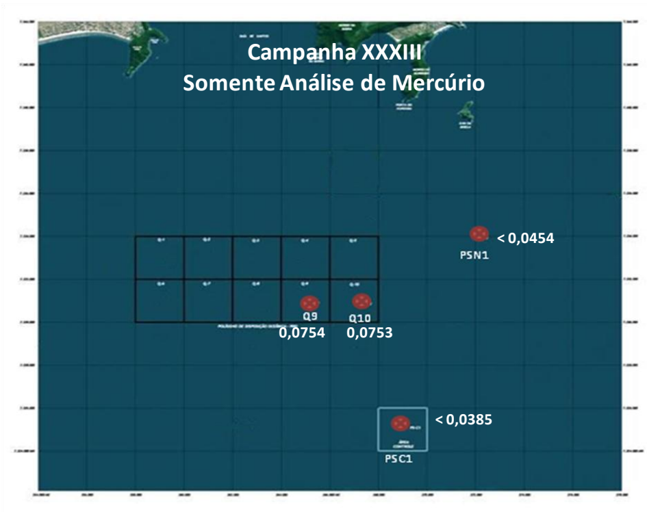
Figura 17.4.5-34. Variação espacial das concentrações de mercúrio, das 4 amostras coletadas durante a Campanha XXXIII, realizada no dia 05 de setembro de 2011.
