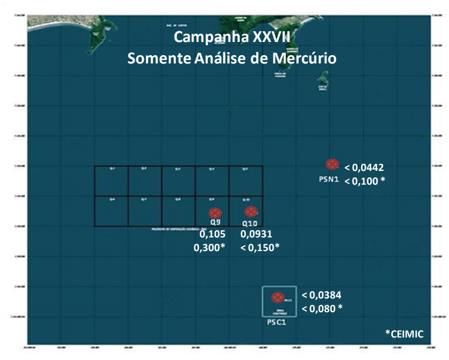
Figura 17.4.5-28. Variação espacial das concentrações de mercúrio, das 4 amostras coletadas durante a Campanha XXVII, realizada no dia 16 de agosto de 2011.
