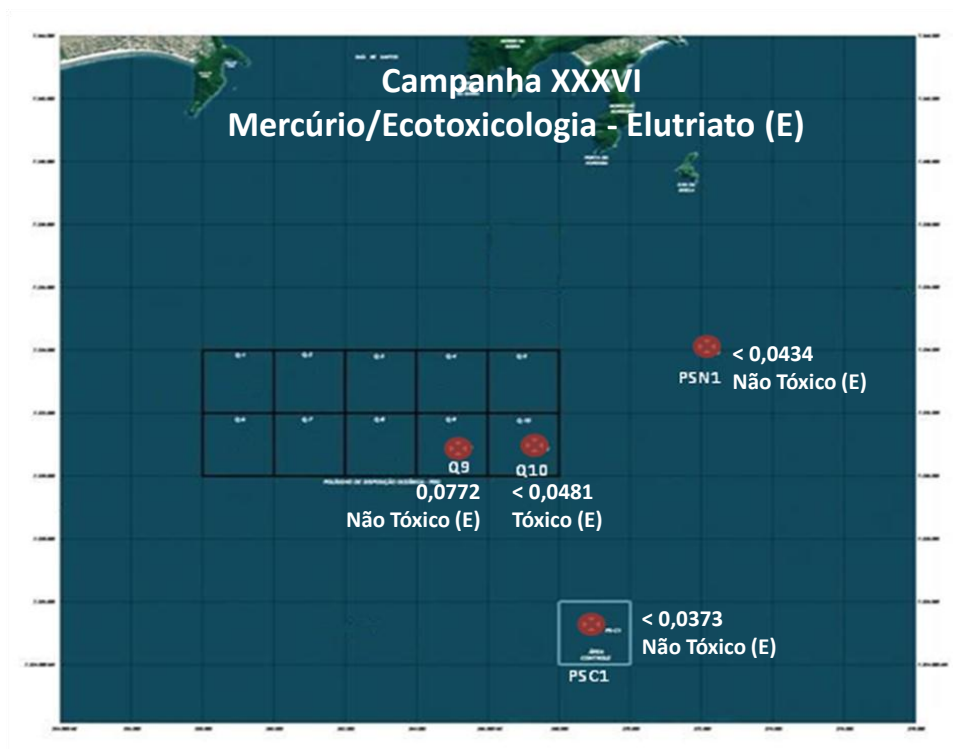
Figura 17.4.5-37. Variação espacial das concentrações de mercúrio e resultados dos ensaios ecotoxicológicos no elutriato, das 4 amostras coletadas durante a Campanha XXXVI, realizada no dia 07 de outubro de 2011.
