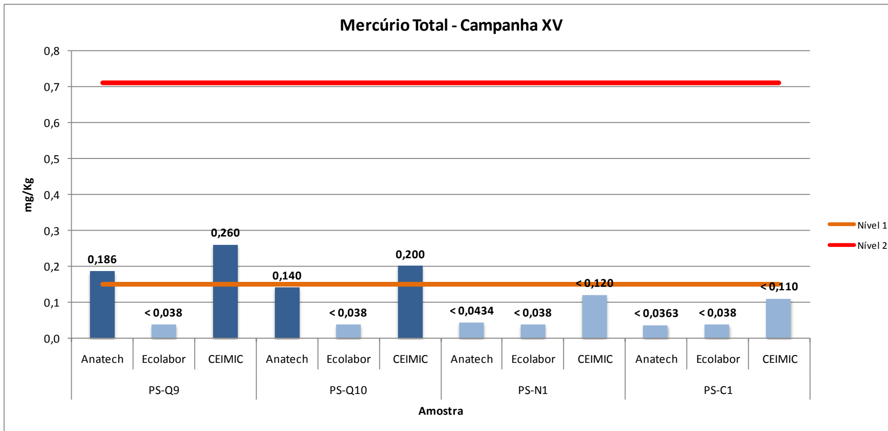
Figura 17.4.1.1-2. Concentração de mercúrio nas amostras de sedimentos coletadas nos pontos PS-Q9, PS-Q10, PS-N1 e PS-C1 da Campanha XV, obtidas pelos laboratórios Anatech (Analytical Technology), Ecolabor e CEIMIC.
