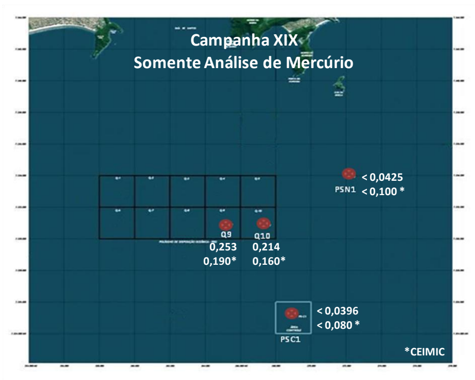
Figura 17.4.5-20. Variação espacial das concentrações de mercúrio, das 4 amostras coletadas durante a Campanha XIX, realizada no dia 19 de julho de 2011.
