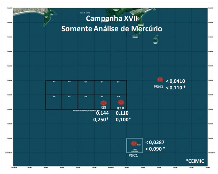
Figura 17.4.5-18. Variação espacial das concentrações de mercúrio, das 4 amostras coletadas durante a Campanha XVII, realizada no dia 12 de julho de 2011.
