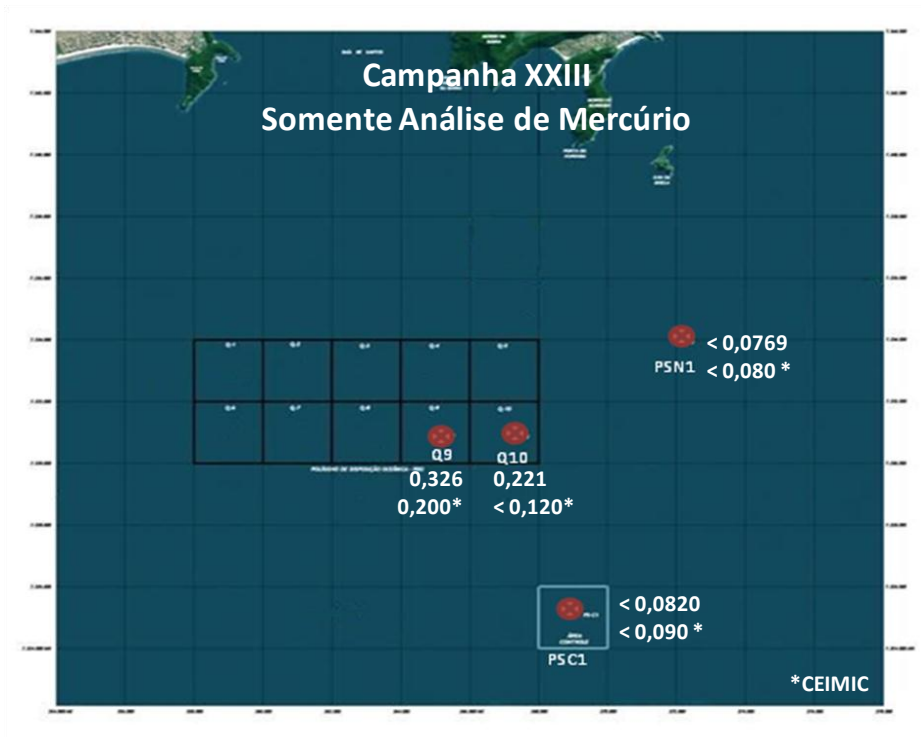
Figura 17.4.5-24. Variação espacial das concentrações de mercúrio, das 4 amostras coletadas durante a Campanha XXIII, realizada no dia 02 de agosto de 2011.
