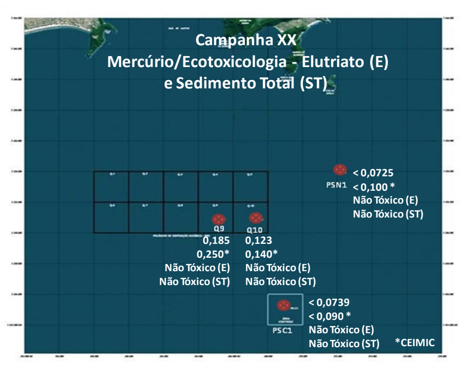
Figura 17.4.5-21. Variação espacial das concentrações de mercúrio e resultados dos ensaios ecotoxicológicos no elutriato e no sedimento total, das 4 amostras coletadas durante a Campanha XX, realizada no dia 22 de julho de 2011.
