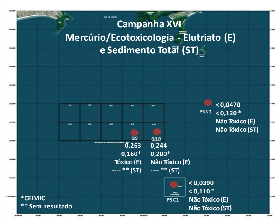
Figura 17.4.5-17. Variação espacial das concentrações de mercúrio e resultados dos ensaios ecotoxicológicos no elutriato e no sedimento total, das 4 amostras coletadas durante a Campanha XVI, realizada no dia 08 de julho de 2011.
