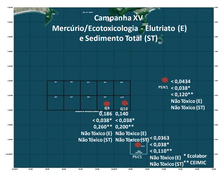
Figura 17.4.5-16. Variação espacial das concentrações de mercúrio e resultados dos ensaios ecotoxicológicos no elutriato e no sedimento total, das 4 amostras coletadas durante a Campanha XV, realizada no dia 30 de junho de 2011.
