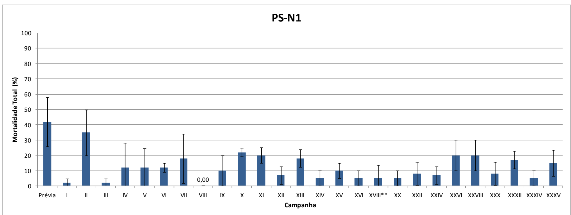
Figura 17.4.4-3. Mortalidade total ( Leptocheirus plumulosus ), com seus respectivos desvios-padrão, encontrada para a amostra coletada em PS-N1 das campanhas cujos resultados foram liberados até o momento. **Resultado dos ensaios ecotoxicológicos das amostras do PBA 17 Mensal.
