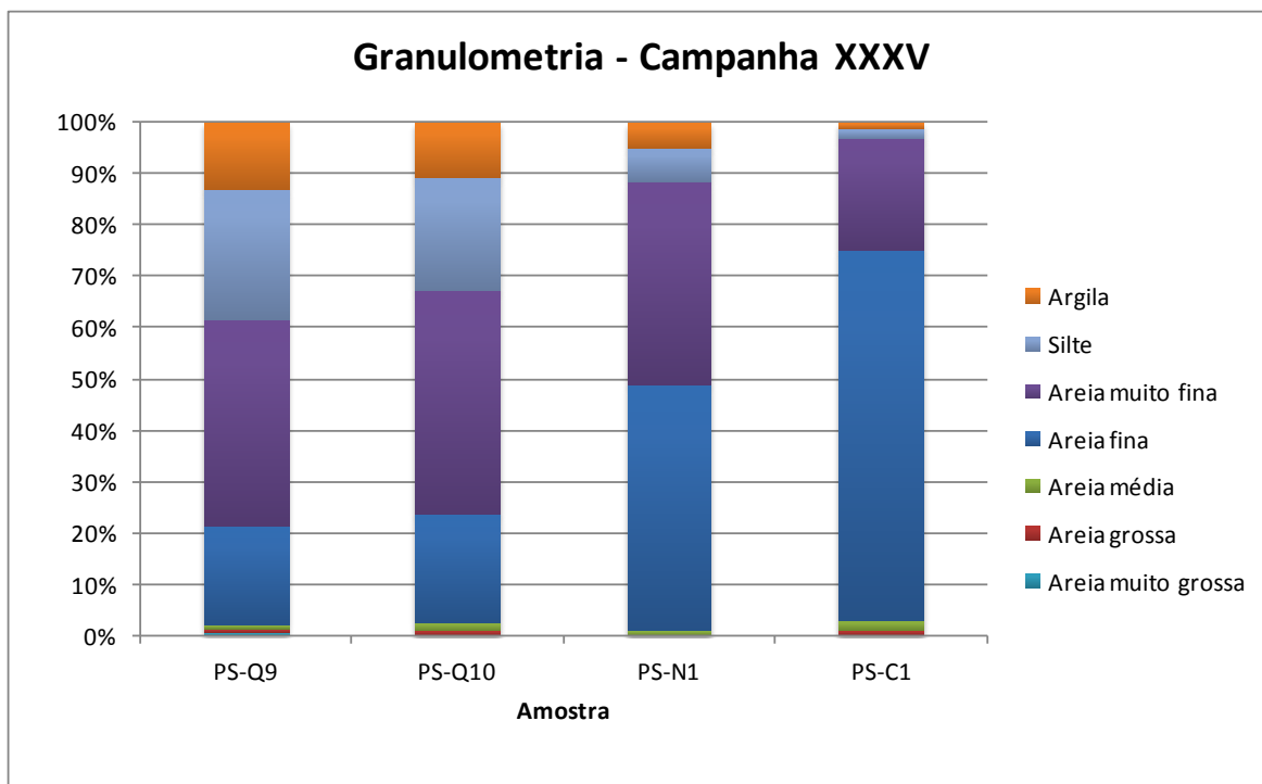
Figura 17.4.2-15. Composição granulométrica do sedimento das amostras PS-Q9, PS-Q10, PS-N1 e PS-C1 da Campanha XXXV.
