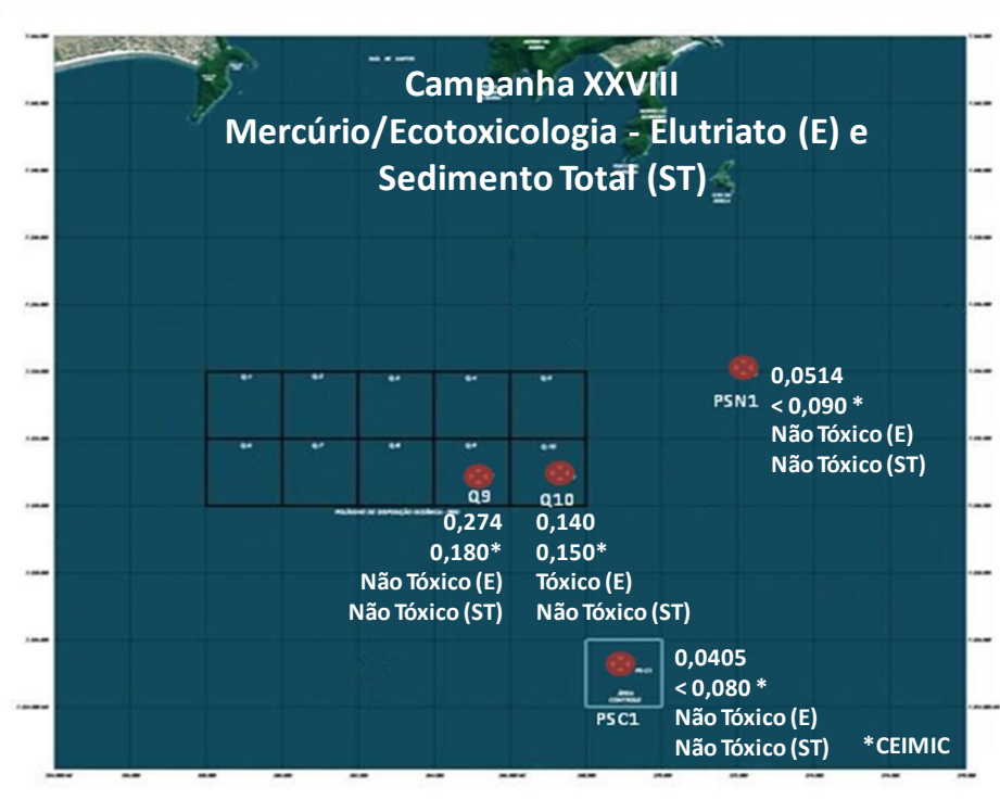
Figura 17.4.5-29. Variação espacial das concentrações de mercúrio e resultados dos ensaios ecotoxicológicos no elutriato e sedimento total, das 4 amostras coletadas durante a Campanha XXVIII, realizada no dia 19 de agosto de 2011.
