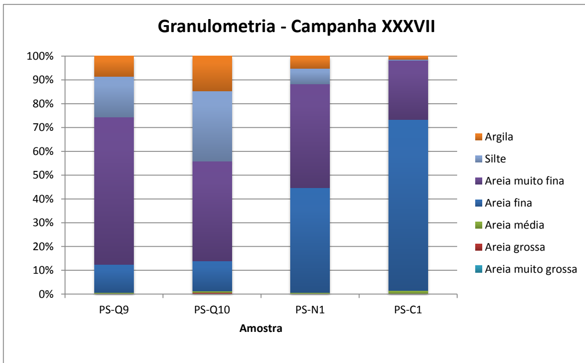
Figura 17.4.2-17. Composição granulométrica do sedimento das amostras PS-Q9, PS-Q10, PS-N1 e PS-C1 da Campanha XXXVII.
