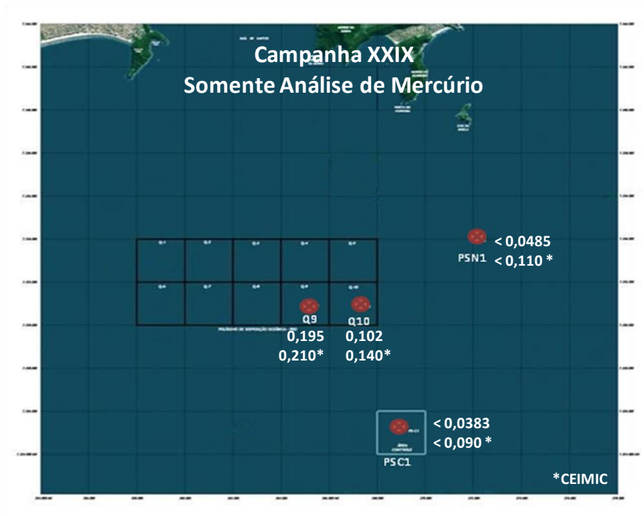
Figura 17.4.5-30. Variação espacial das concentrações de mercúrio, das 4 amostras coletadas durante a Campanha XXIX, realizada no dia 23 de agosto de 2011.
