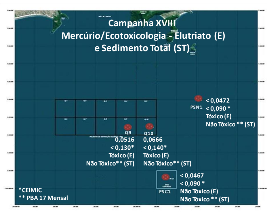
Figura 17.4.5-19. Variação espacial das concentrações de mercúrio e resultados dos ensaios ecotoxicológicos no elutriato e no sedimento total, das 4 amostras coletadas durante a Campanha XVIII, realizada no dia 15 de julho de 2011.
