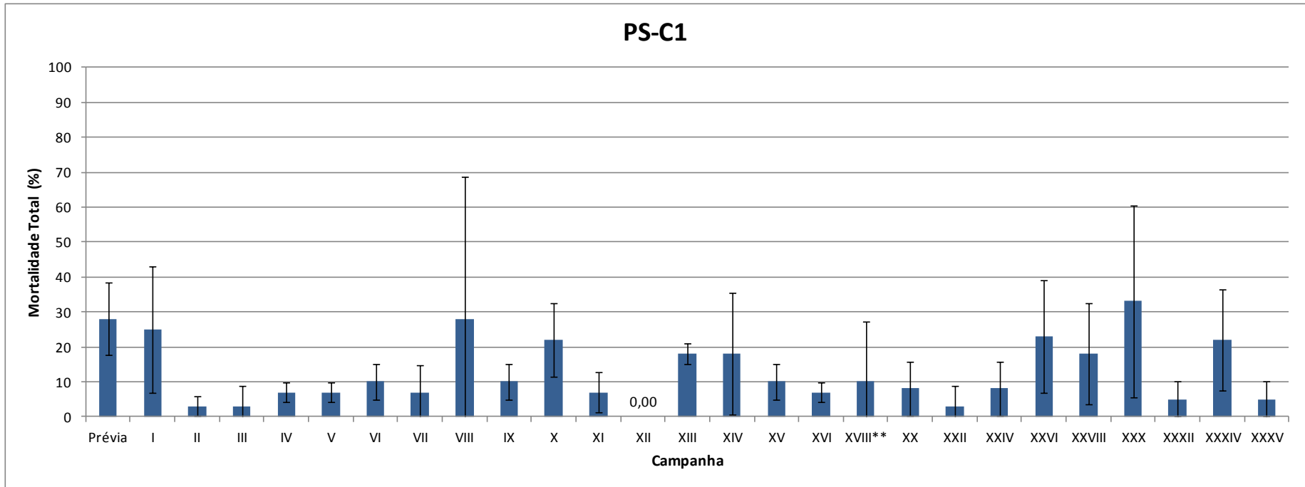
Figura 17.4.4-4. Mortalidade total ( L. plumulosus ), com seus respectivos desvios-padrão, encontrada para a amostra coletada em PS-C1 das campanhas cujos resultados foram liberados até o momento.**Resultado dos ensaios ecotoxicológicos das amostras do PBA 17 Mensal.
