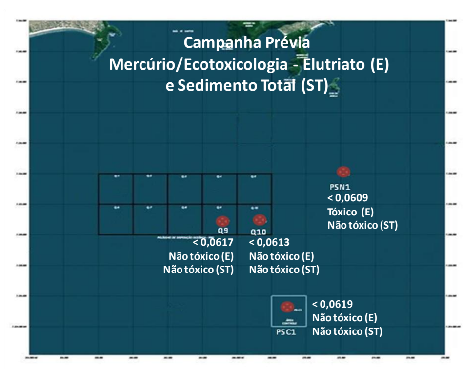
Figura 17.4.5-1. Variação espacial das concentrações de mercúrio e resultados dos ensaios ecotoxicológicos no elutriato e no sedimento total, das 4 amostras coletadas durante a Campanha Prévia, realizada no dia 3 de fevereiro de 2011.
