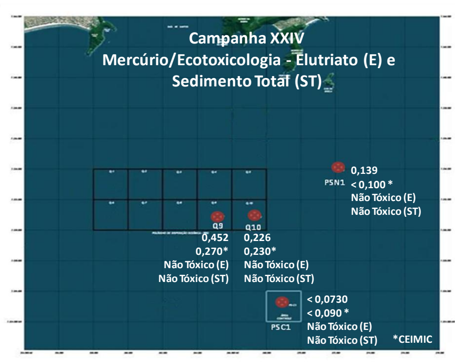
Figura 17.4.5-25. Variação espacial das concentrações de mercúrio e resultados dos ensaios ecotoxicológicos no elutriato e no sedimento total, das 4 amostras coletadas durante a Campanha XXIV, realizada no dia 05 de agosto de 2011.
