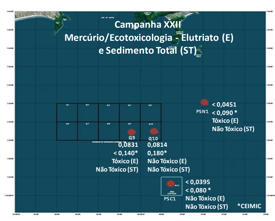
Figura 17.4.5-23. Variação espacial das concentrações de mercúrio e resultados dos ensaios ecotoxicológicos no elutriato e no sedimento total, das 4 amostras coletadas durante a Campanha XXII, realizada no dia 29 de julho de 2011.
