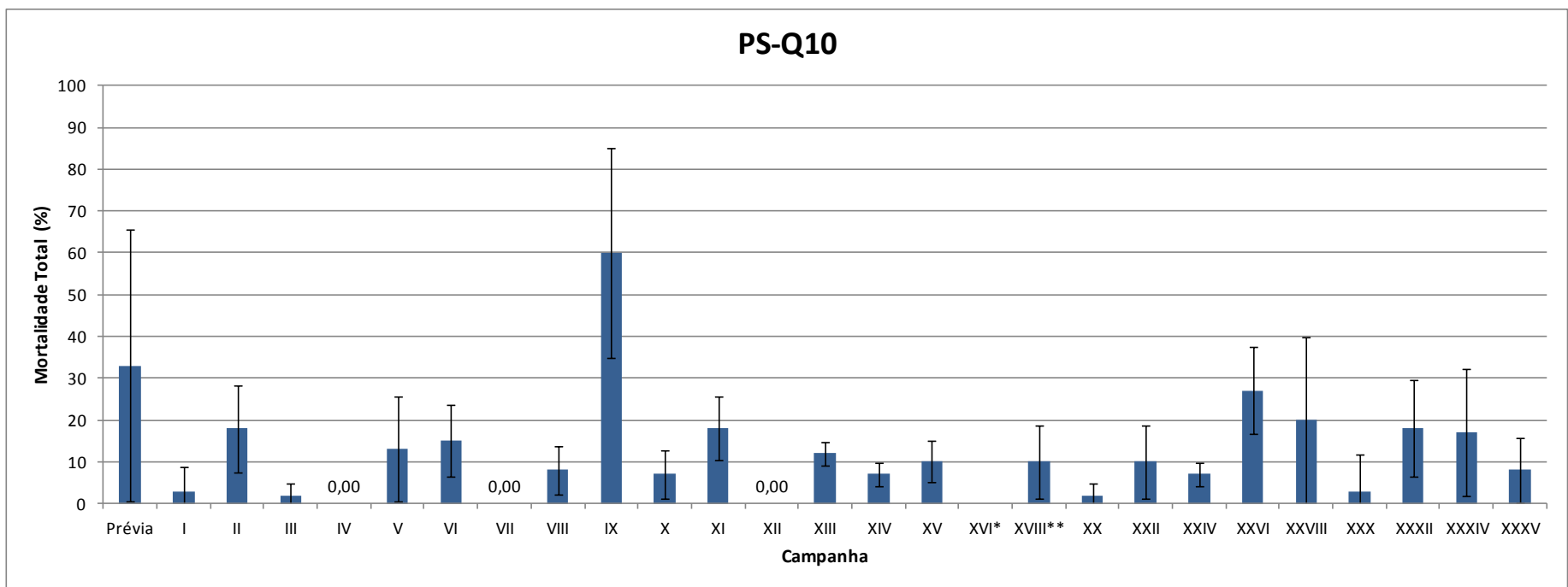
Figura 17.4.4-2. Mortalidade total ( Leptocheirus plumulosus ), com seus respectivos desvios-padrão, encontrada para a amostra coletada em PS-Q10 das campanhas cujos resultados foram liberados até o momento. *Amostras cujo ensaio não foi realizado, devido à falta do organismo teste. **Resultado dos ensaios ecotoxicológicos das amostras do PBA 17 Mensal.
