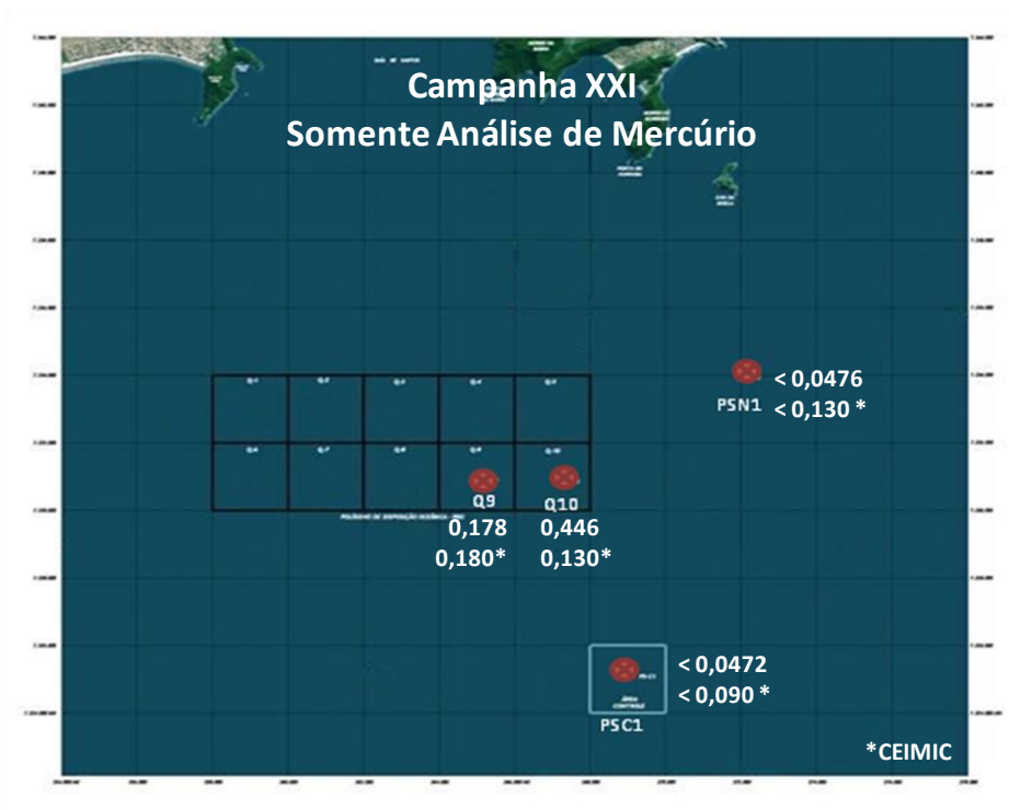
Figura 17.4.5-22. Variação espacial das concentrações de mercúrio, das 4 amostras coletadas durante a Campanha XXI, realizada no dia 26 de julho de 2011.
