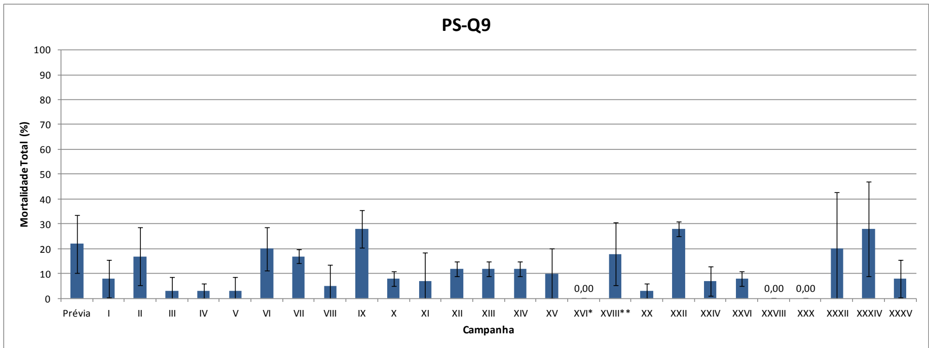
Figura 17.4.4-1. Mortalidade total ( Leptocheirus plumulosus ), com seus respectivos desvios-padrão, encontrada para a amostra coletada em PS-Q9 das campanhas cujos resultados foram liberados até o momento. *Amostras cujo ensaio não foi realizado, devido à falta do organismo teste. **Resultado dos ensaios ecotoxicológicos das amostras do PBA 17 Mensal.
