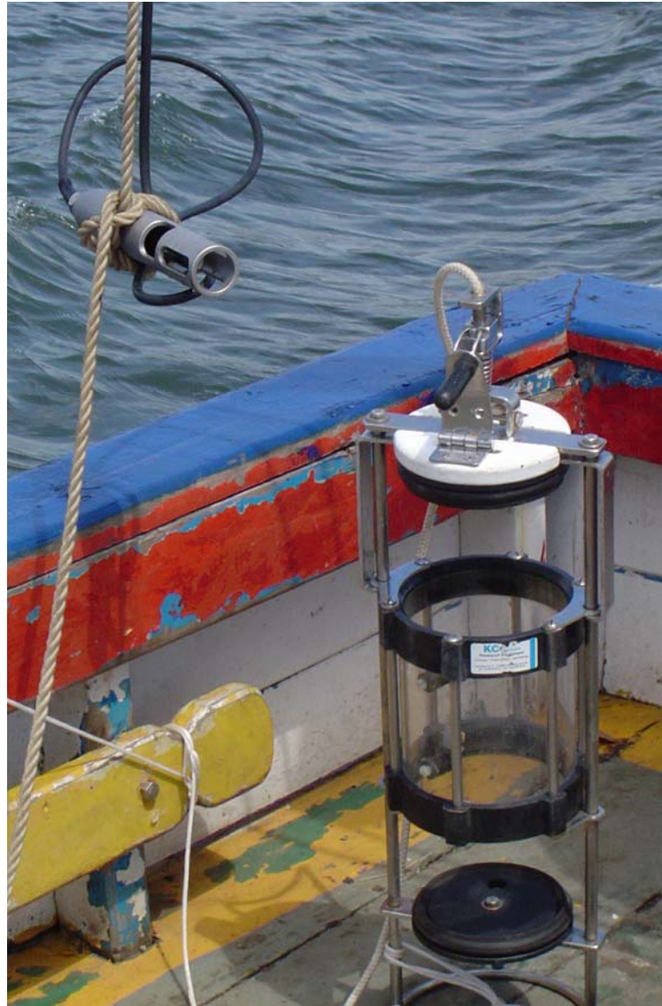
Vista do sensor do Termosalinômetro e do Coletor D'água
