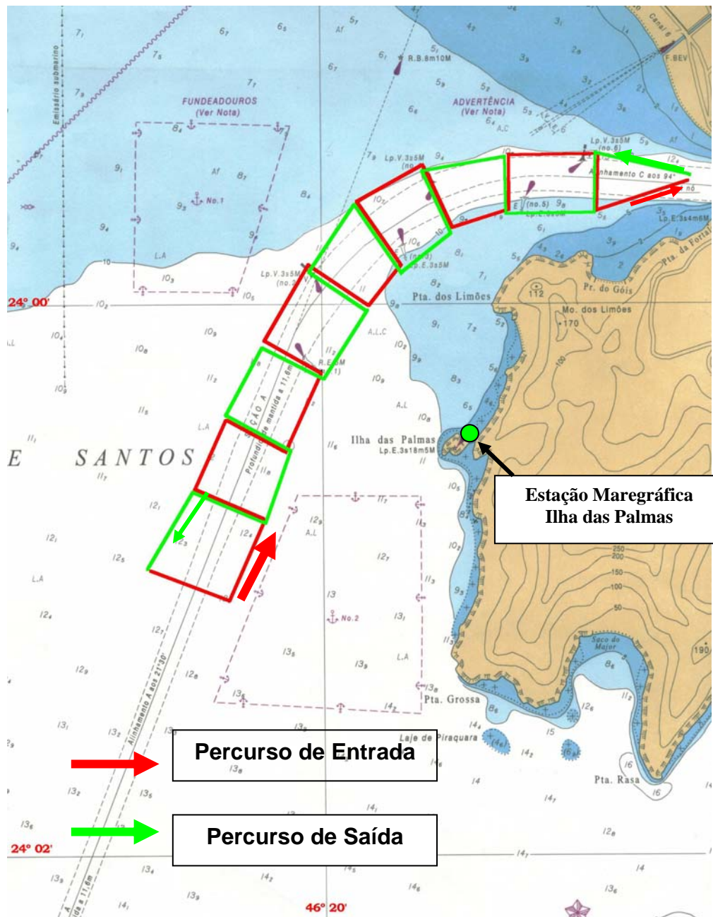
Fig. 1- Percurso realizado nas medições com ADCP na área oceânica
